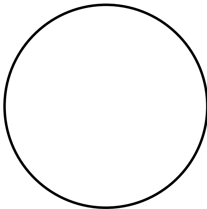
Uranus Blue
